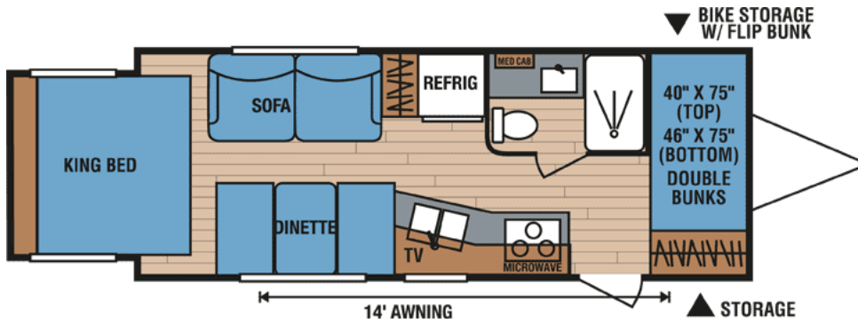
KZ Spree 220KS
